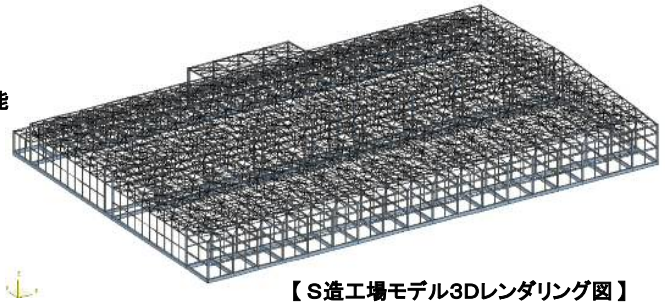
【S造工場モデル3Dレンダリング図】
