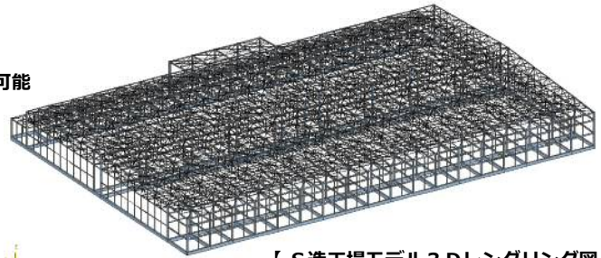
【S造工場モデル3Dレンダリング図】
