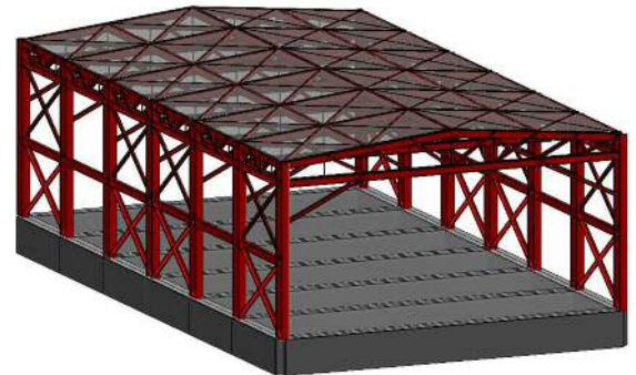
【S造モデル CREA Viewer レンダリング図】
