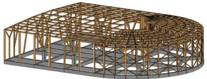
【木造+RC造モデル CREAViewer レンダリング図】
